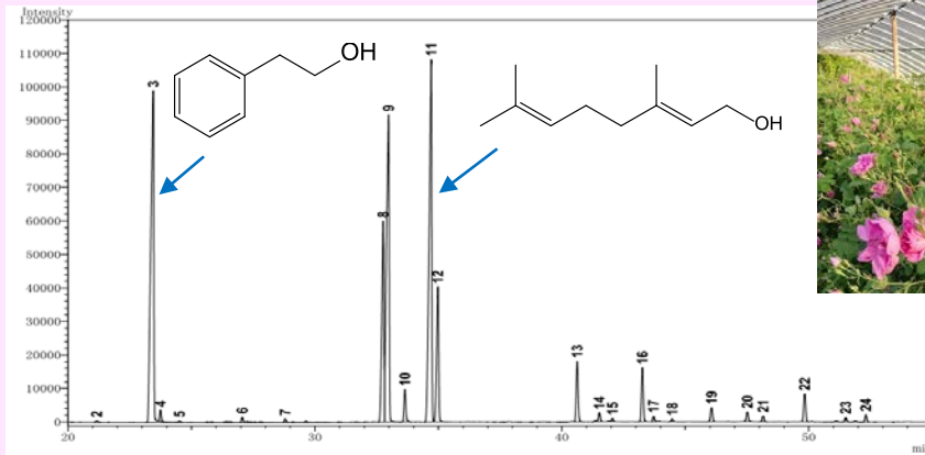
ローズオイルのガスクロマトグラフ分析結果
