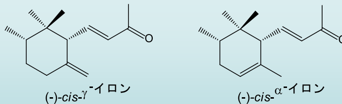
香気物質イロンの分子構造
