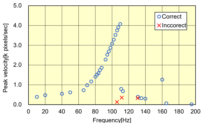
図3 周波数応答特性
