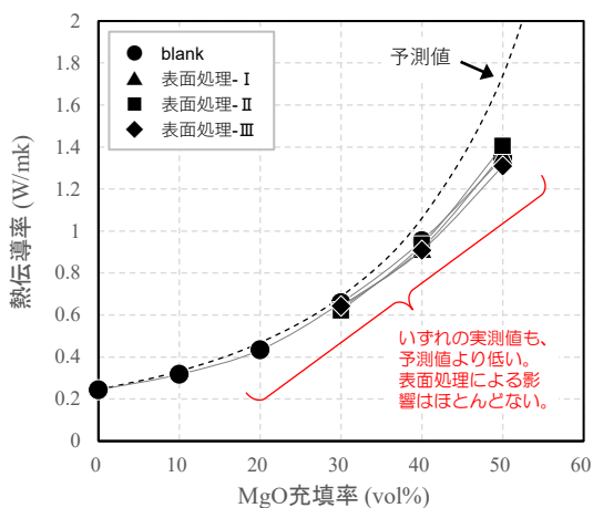
複合材の熱伝導性評価(平均粒径20 μm)
