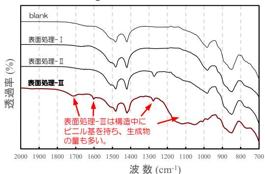
MgOのFT-IRスペクトル
