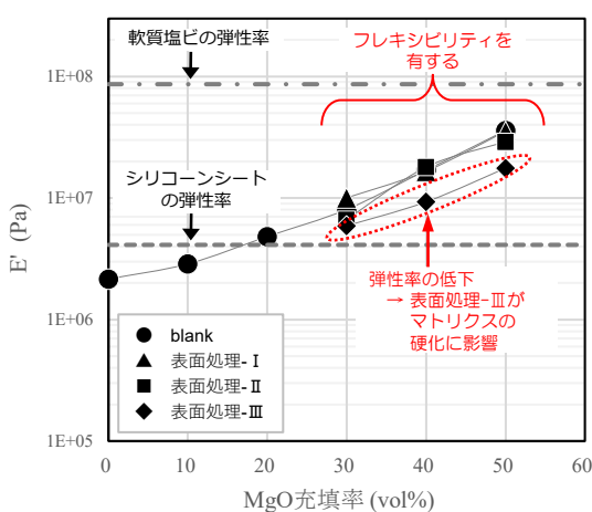
複合材のフレキシビリティ評価(平均粒径20 μm)
