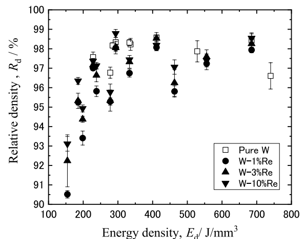
図 1 W-Re 造形体の相対密度とエネルギー密度の関係
